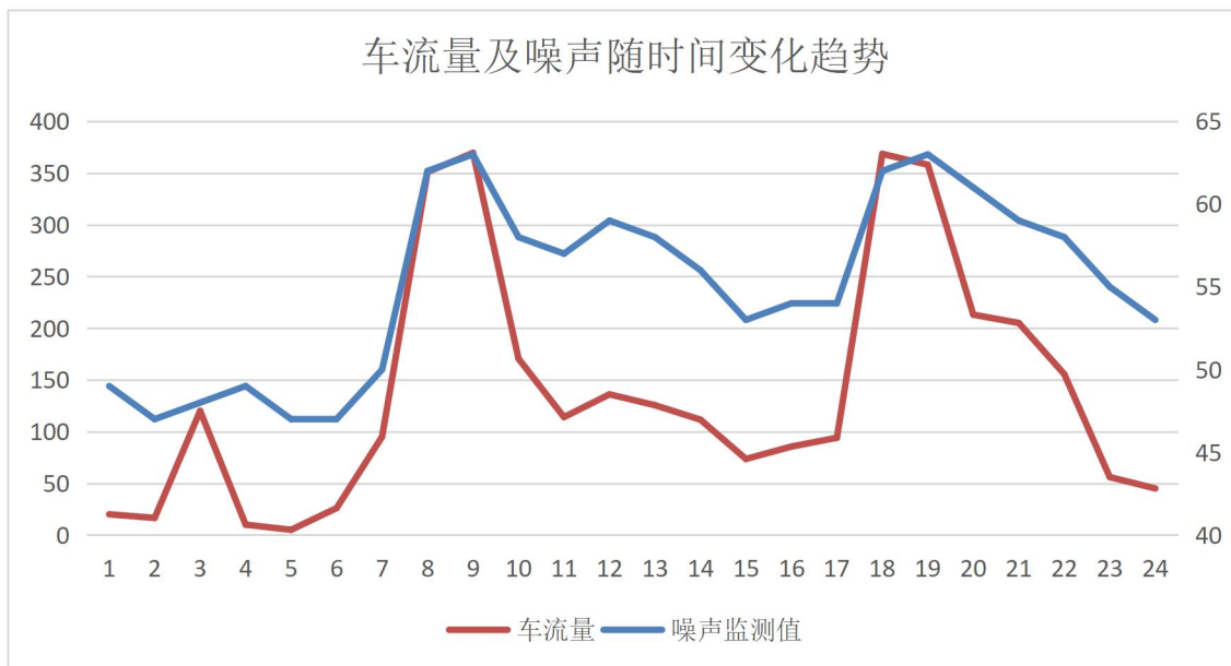
图8.4-3 声级和总车流量随时间变化趋势
