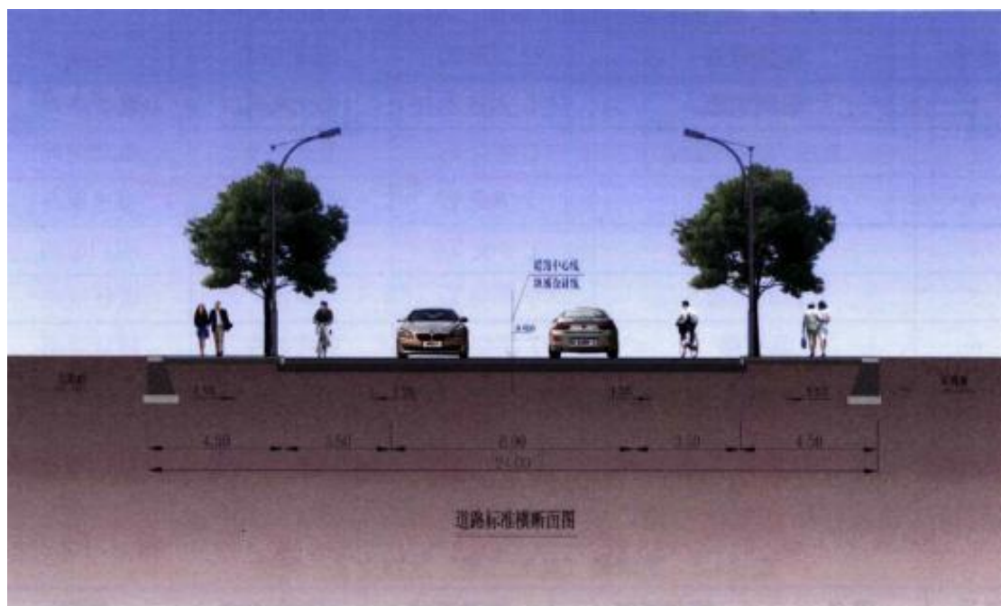
图 2.2-3 下湾路西段
